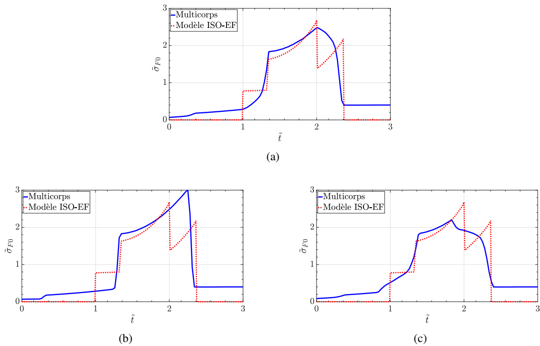
FIGURE 4 – Évolution de la contrainte en pied de dent maximale adimensionnée \tilde{\sigma}_{F0} au cours de l’engrènement pour une des dents de la roue menante au couple adimensionné \tilde{C} = 0,90 (a), puis à \tilde{C} = 0,25 (b), et enfin pour \tilde{C} = 2,2 (c).
